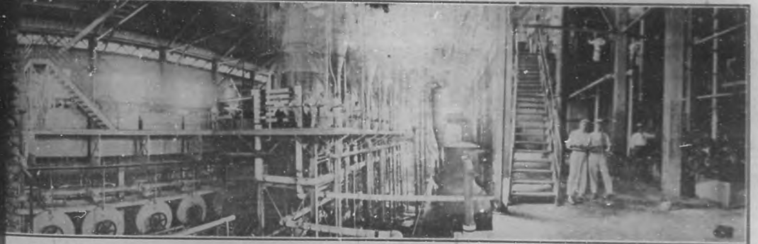
MAQUINAS DEL INGENIO.—CENTRIFUGAS, PESAS AUTOMATICAS, ROMANAS Y EL ALMACEN DE AZUCAR
